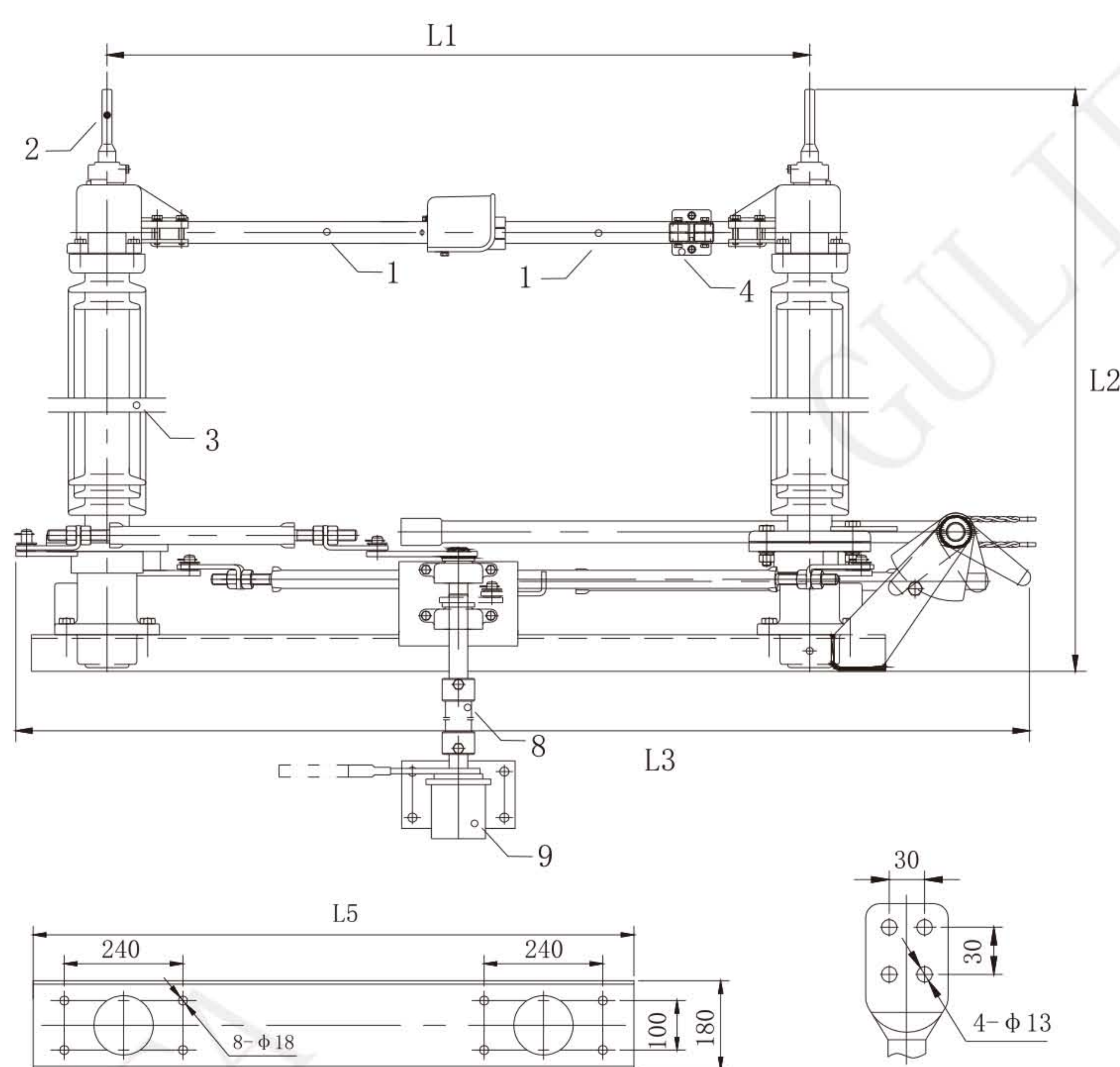
接线板尺寸
