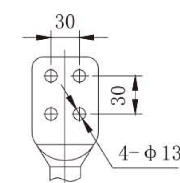
接线板尺寸
